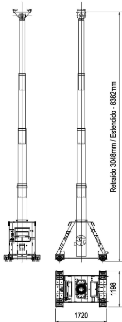
Pórtico Hidráulico de 400t
