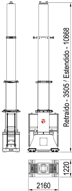
Pórtico Hidráulico de 500t - 10.60m
